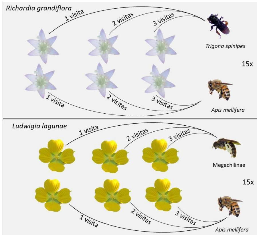
Fig 2. Esquema dos tratamentos adotados em cada grupo (abelhas nativas e Apis mellifera ). Richardia grandiflora e Ludwigia lagunae recebendo uma, duas e três visitas de cada espécie de abelha. Os tratamentos foram repetidos 15 vezes para cada espécie de planta.
