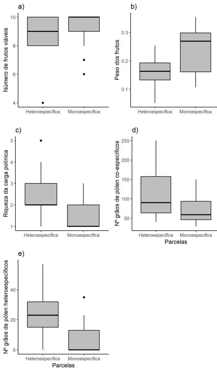
Figura 2. Relação entre as variáveis e o tipo de parcela (Heteroespecífica e Monoespecífica), a- número de frutos viáveis ( p < 0.006 ), b- peso dos frutos ( p < 0.731 ), riqueza da carga polínica ( p < 0.0006 ), d- número de grãos de pólen co-específicos ( p < 0.612 ) e, e- número de grãos de pólen heteroespecíficos ( p < 0.0001 ) em parcelas mono e heteroespecíficas de Richardia grandiflora . As variáveis representadas no eixo Y foram transformados para \log_{10} , de modo a melhorar o ajuste do modelo.
