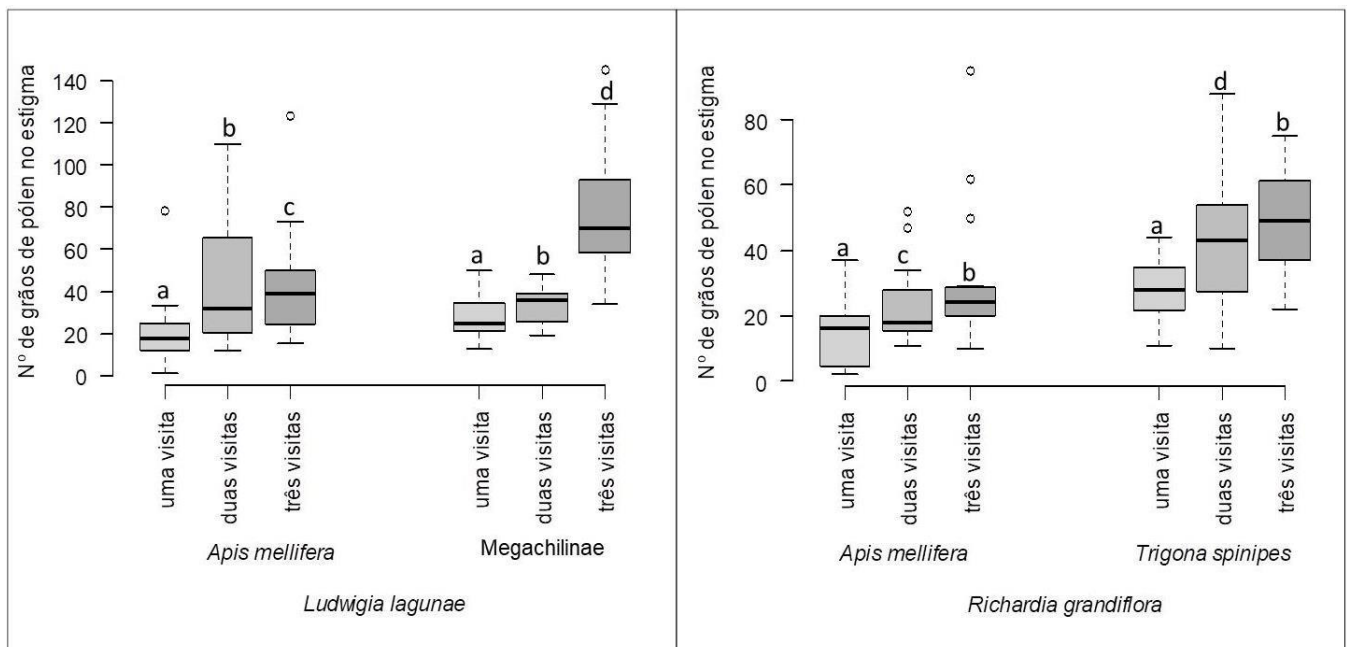
Fig 3. Quantidade de grãos de pólen depositados no estigma das flores de Ludwigia lagunae (gráfico à esquerda) e Richardia grandiflora (gráfico à direita) após uma, duas e três visitas de Apis mellifera e das abelhas nativas Megachilinae e Trigona spinipes . Letras diferentes indicam diferenças entre os tratamentos. Ludwigia lagunae ( p = 0,0286 ) e Richardia grandiflora ( p = 0,0001 ).
