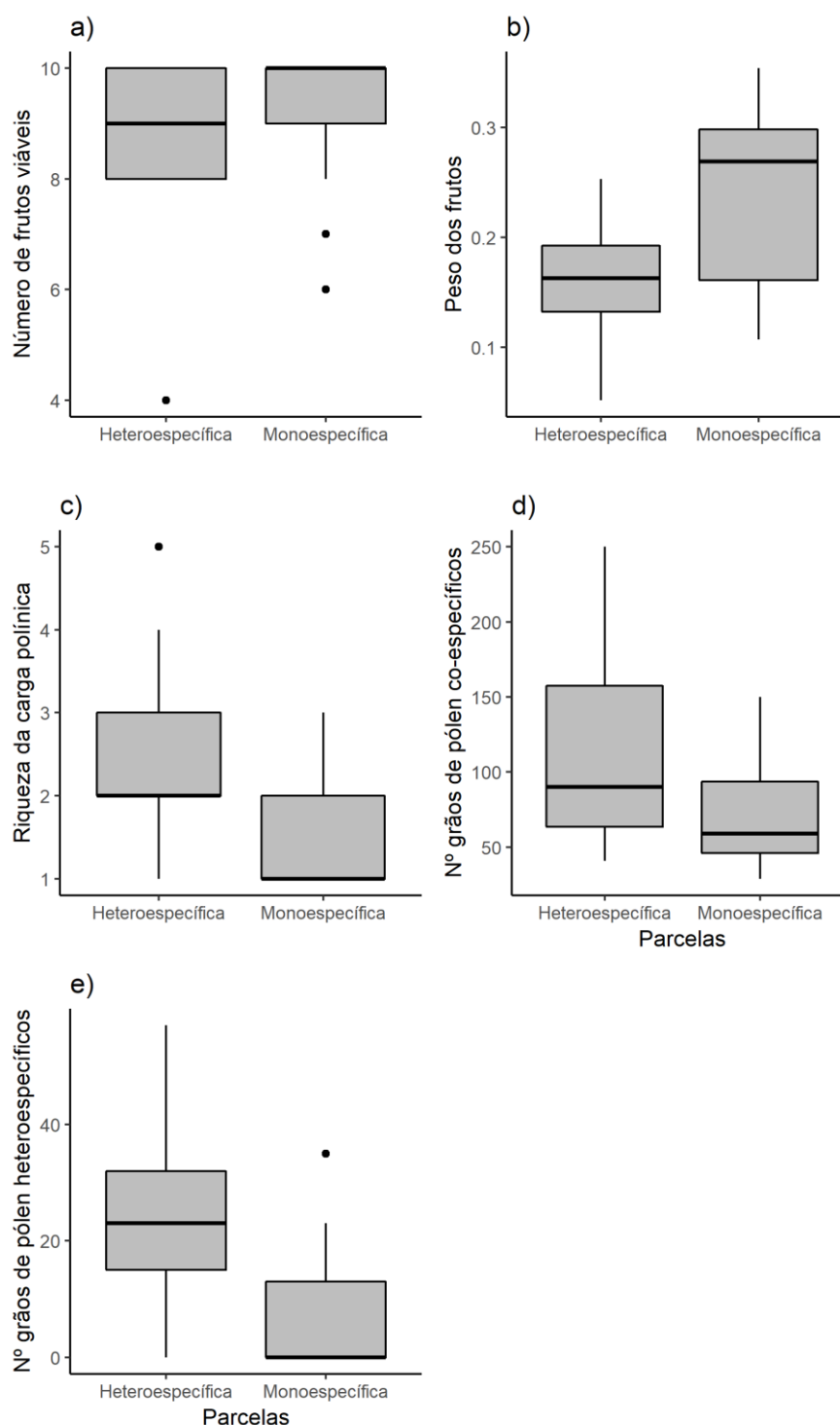
Figura 1. Relação entre as variáveis e o tipo de parcela (Heteroespecífica e Monoespecífica), a- número de frutos viáveis ( p = 0.378 ), b- peso dos frutos ( p < 0.009 ), riqueza da carga polínica ( p < 0.009 ), d- número de grãos de pólen co-específicos ( p < 0.026 ) e, e- número de grãos de pólen heteroespecíficos ( p < 0.003 ) em parcelas mono e heteroespecíficas de Ludwigia lagunae . As variáveis representadas no eixo Y foram transformados para log10, de modo a melhorar o ajuste do modelo.
